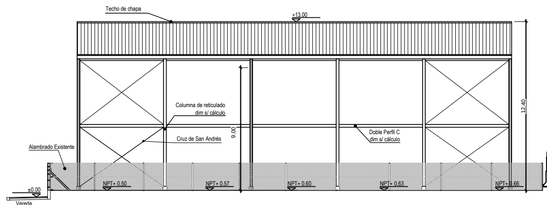
VISTA LATERAL
