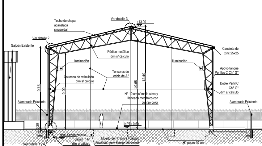
CORTE / VISTA TRANSVERSAL A-A
