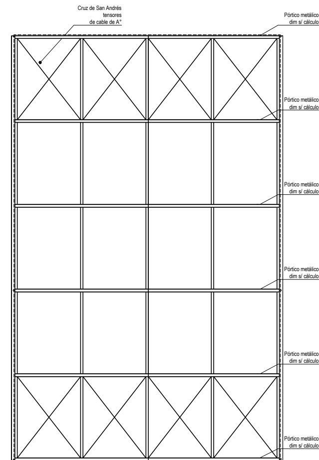
PLANTA DE ESTRUCTURA DE TECHOS
