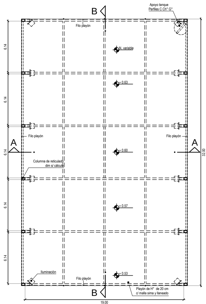
PLANTA
