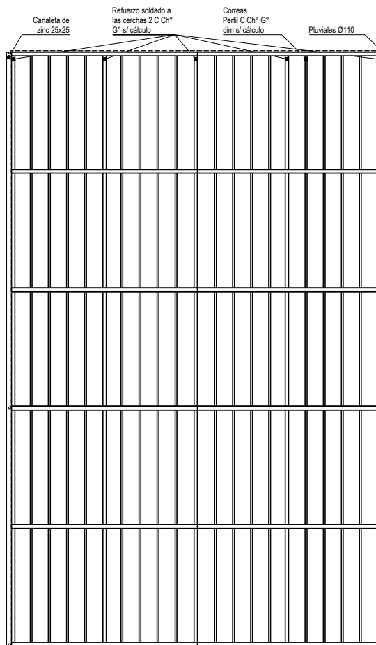
PLANTA DE ESTRUCTURA Y CORREAS
