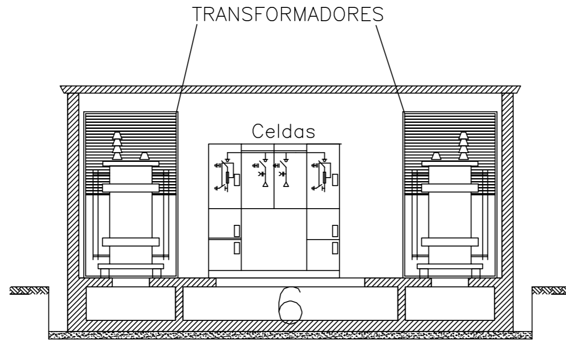
Corte B-B
