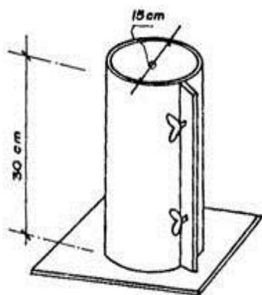
Fig. 8.2 Molde de acero, para elaboración de probetas de ensayo
