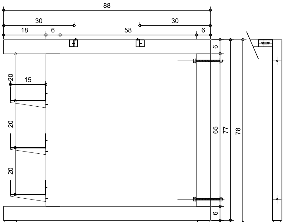
3 Lateral: Estructura metalica para mesa con planchuelas soldadas y regatones plasticos. Bandejas Portacables Perforadas Galv. 150mm
