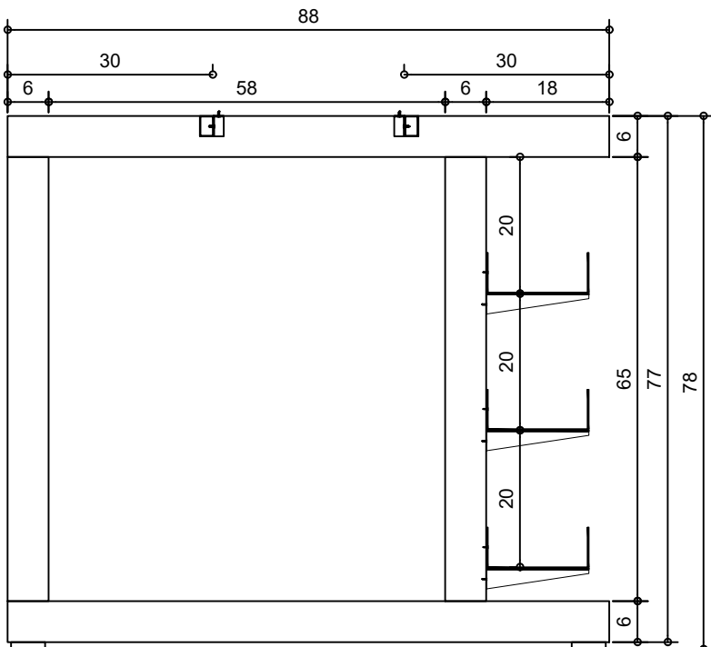
1 Lateral: Estructura metalica para mesa con planchuelas soldadas y regatones plasticos. Bandejas Portacables Perforadas Galv. 150mm
