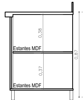
CORTE
