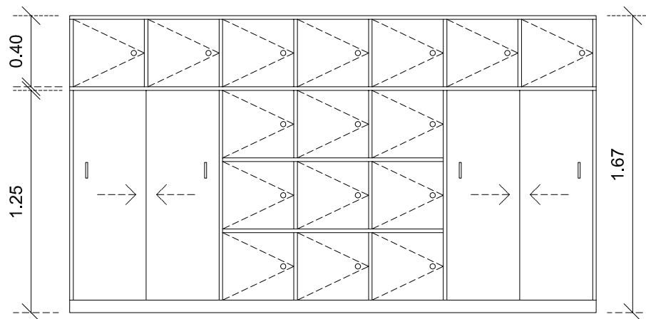
Vista frente
