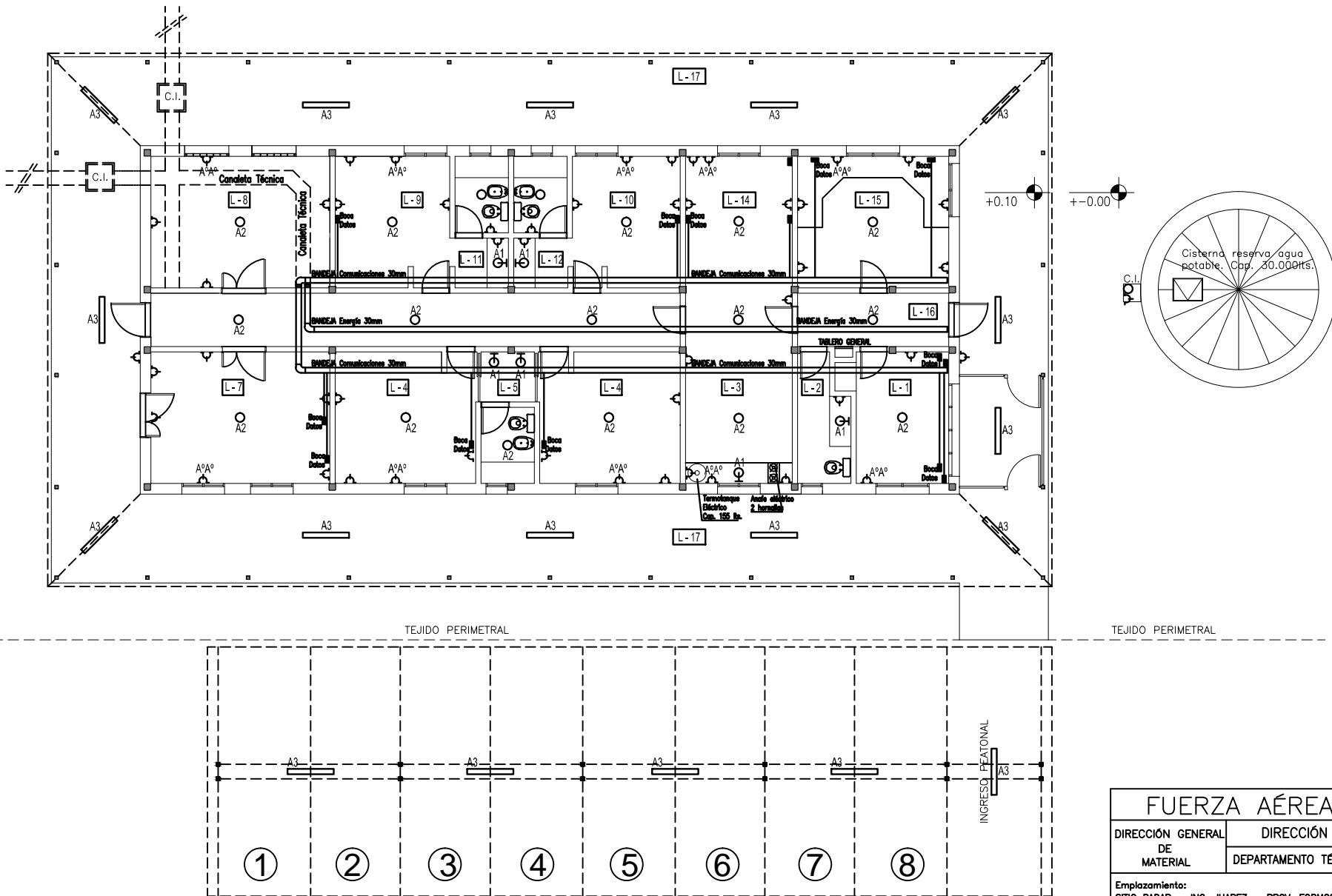
7 PLANTA GENERAL ELECTRICIDAD Escala 1:150
