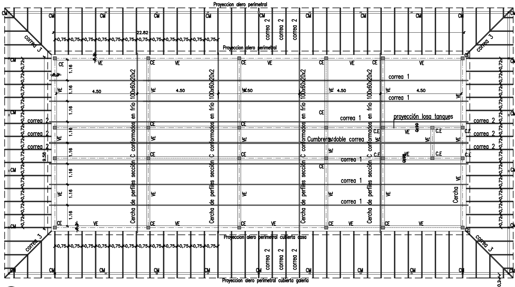
5-a PLANTA ESTRUCTURA DE CUBIERTA Escala 1:120
