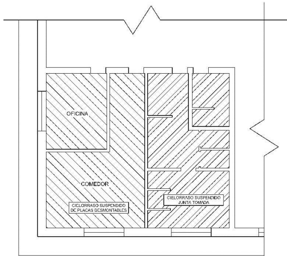
CIELORRASOS SECTOR 1
