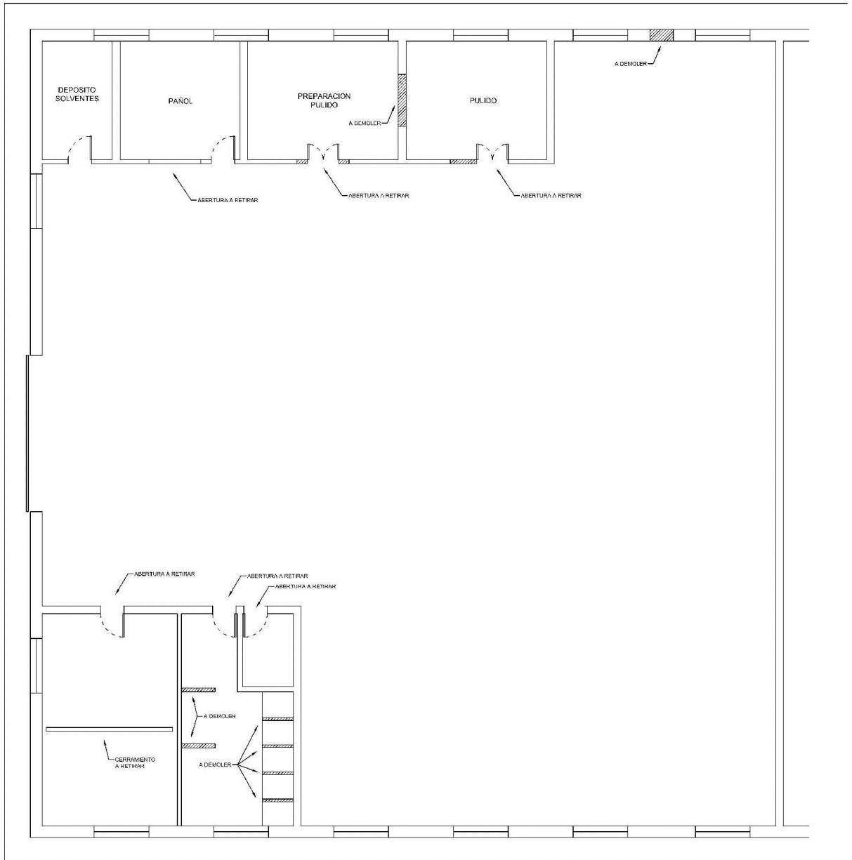
PLANTA DEMOLICION
