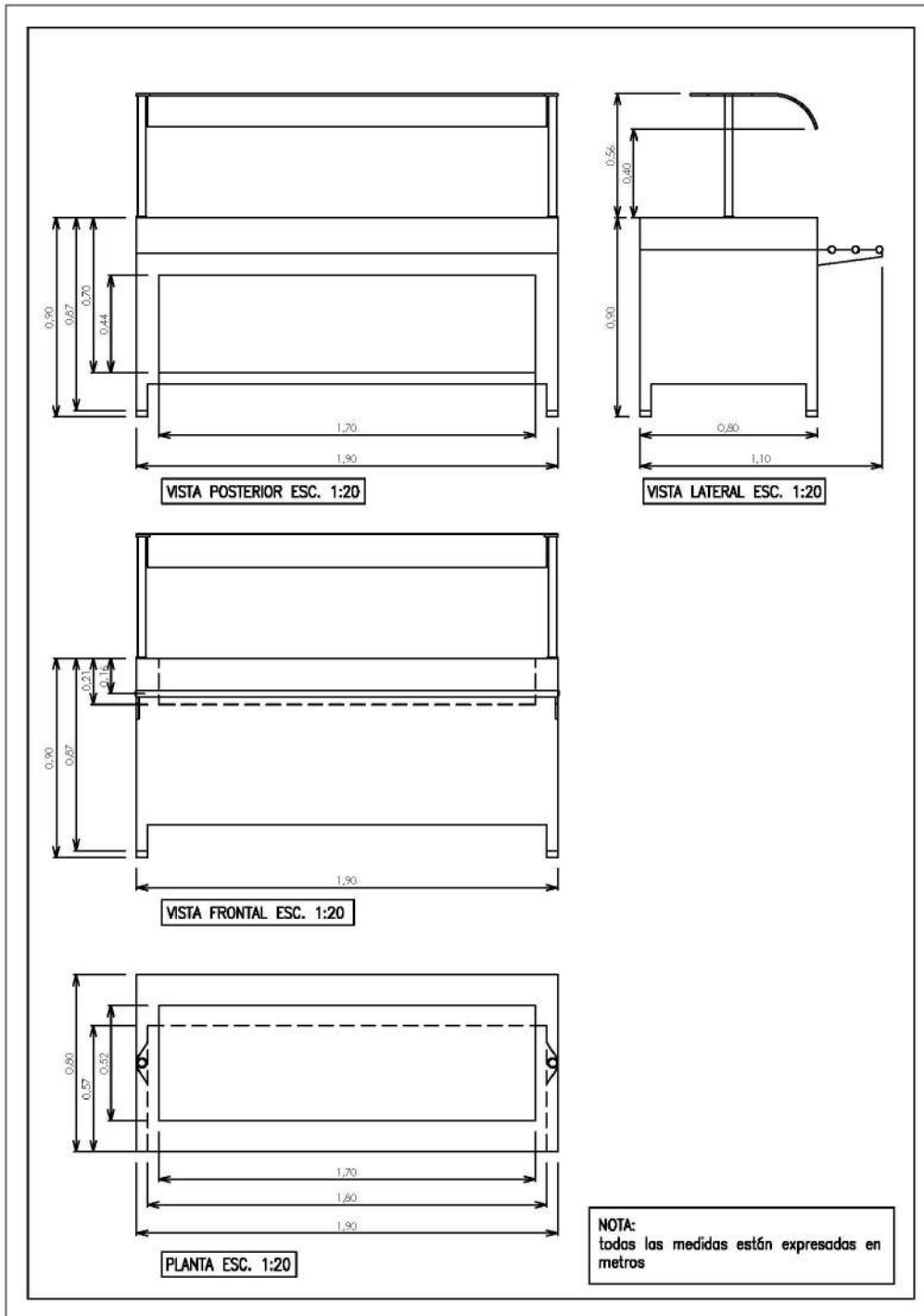
Esquema referencial con dimensiones.
